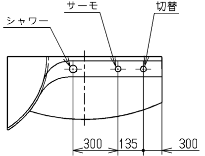
水栓取付け位置（フリー）
