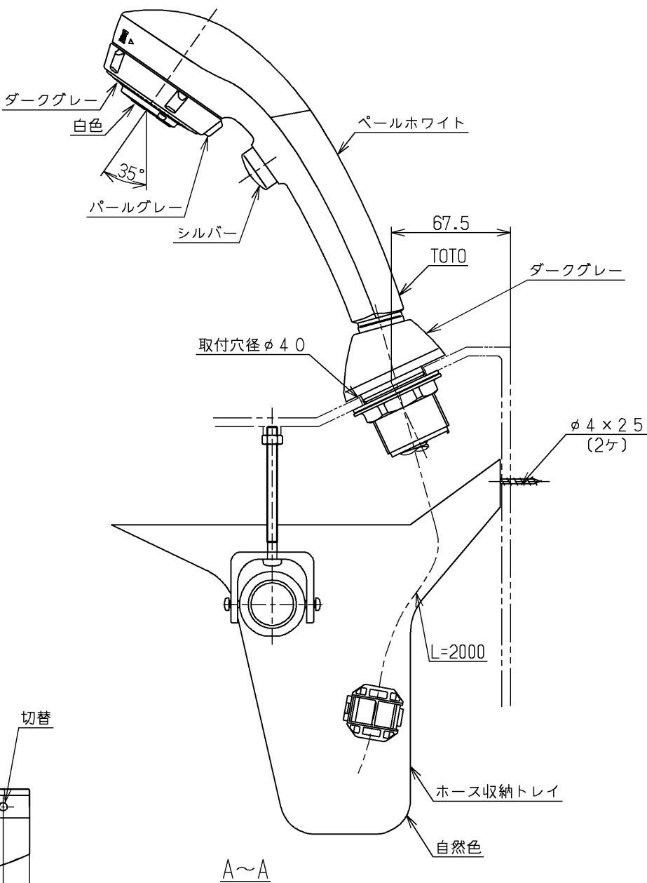
水栓取付け位置（フリー）
